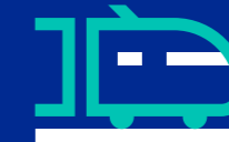
Schienenverkehr
